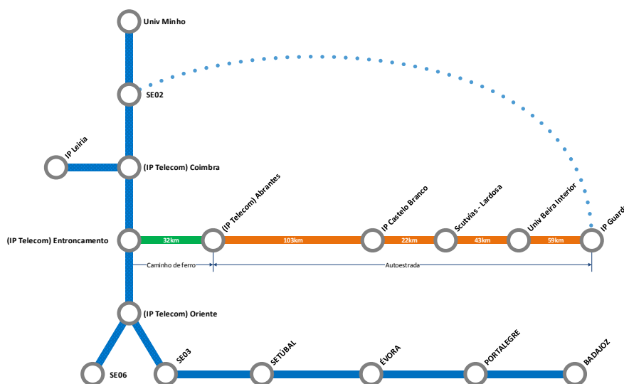
Figura 17 - Serviço de Rede FCCN. Topologia da plataforma de transmissão ótica, 2016
